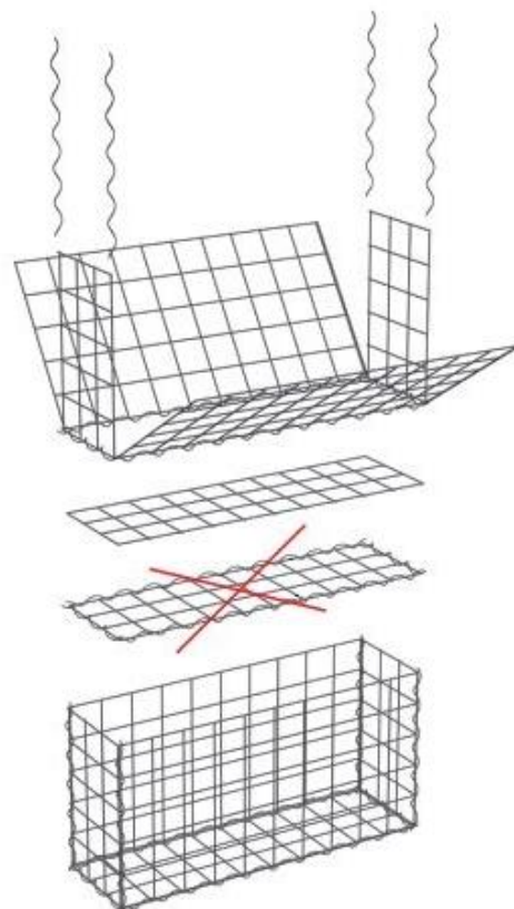
příklad ukládaní košů na sebe
